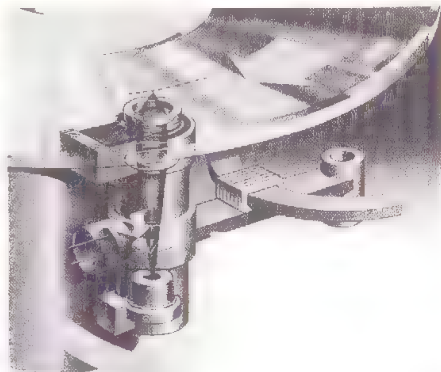
Het in de MF toegepaste Philips Laser pick up mechanisme.
